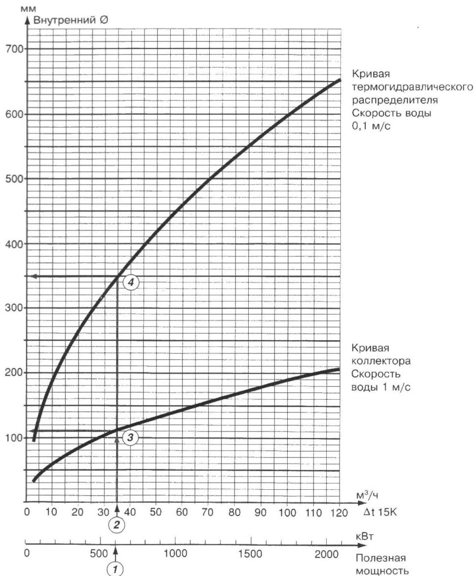
Рисунок 7. График для определения внутреннего диаметра коллекторов
